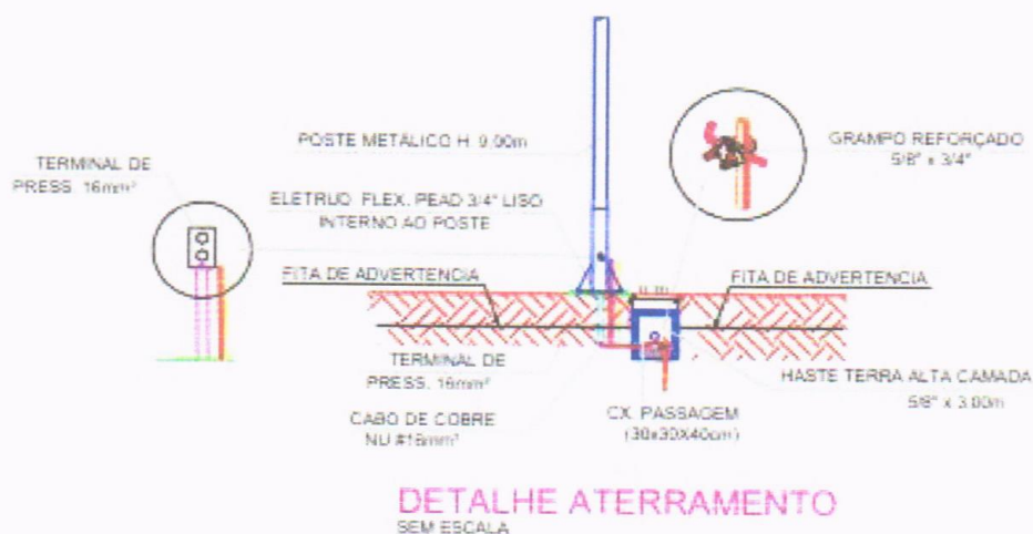
Imagem 04: Detalhe do Aterramento dos postes.
