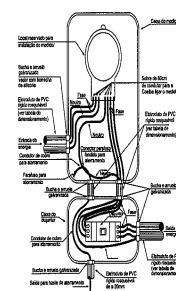
INSTALAÇÃO DE DISJUNTOR - CAIXA PLÁSTICA
